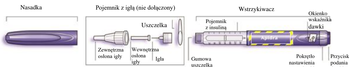
Schemat budowy wstrzykiwacza
